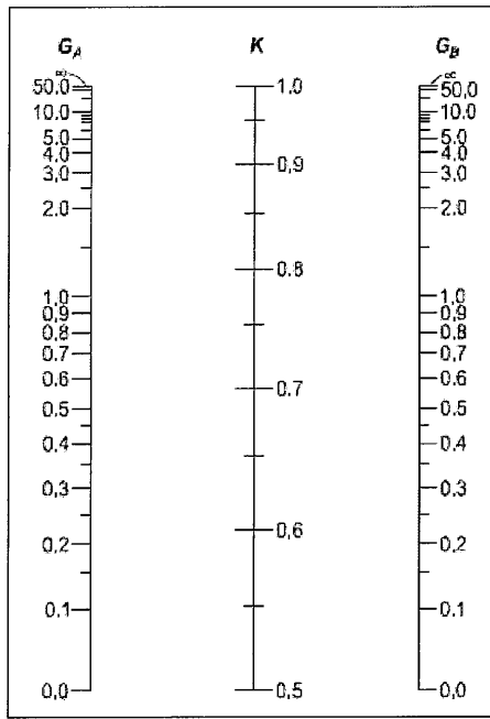
Şekil 6.1 – Yanal yerdeğiřtirmesi önlenmiş sistemlerde burkulma boyu katsayısı, K
