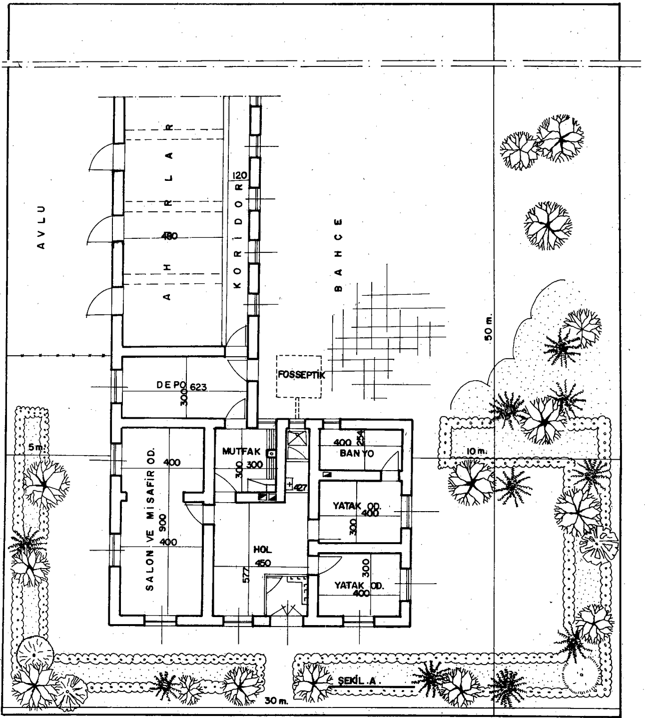
Şekil A — Av ve Ahır Birleşik Planı
