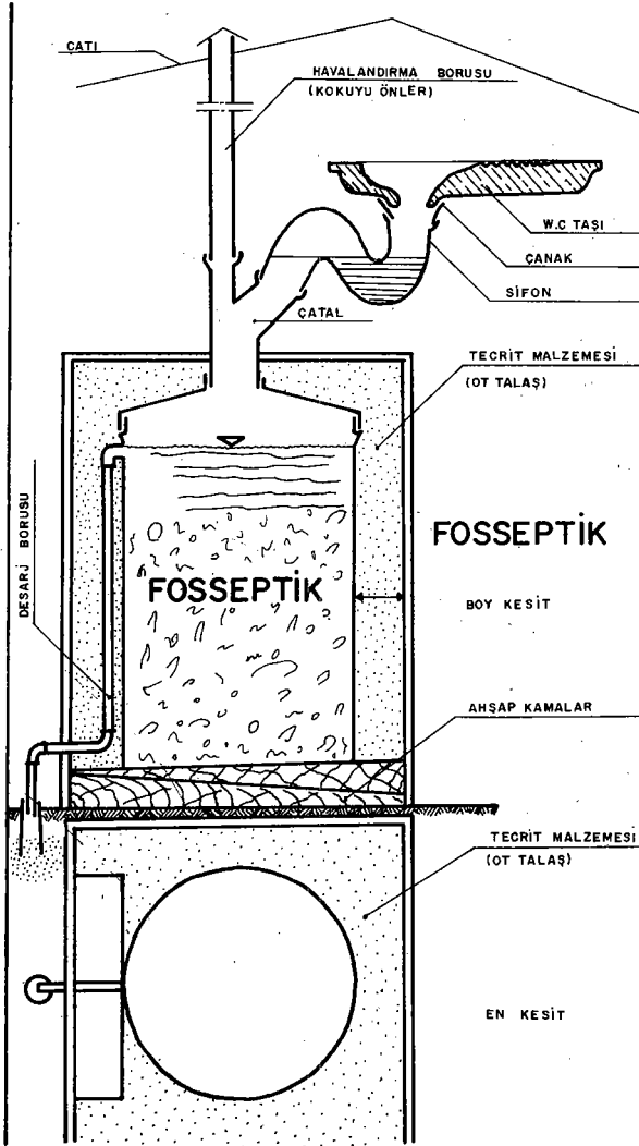
ŞEKİL B — Taşınabilir Fosseptik
