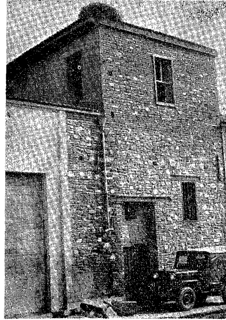
Hatıl bağlantıları mütemadi yapılmayan bir bina
