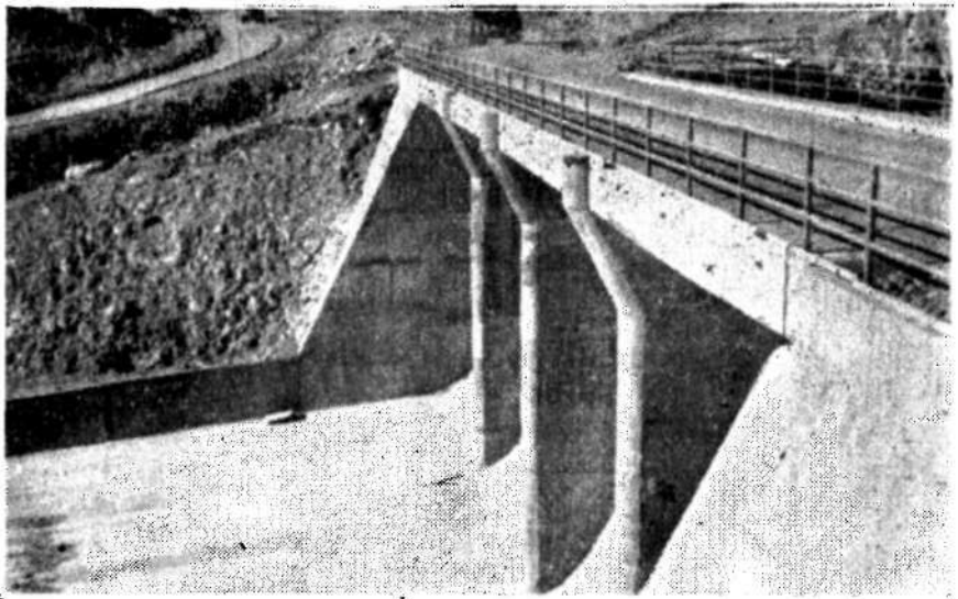
Çubuk II Barajı — Dolu Savak Baraj Tarafından Görüntü.
