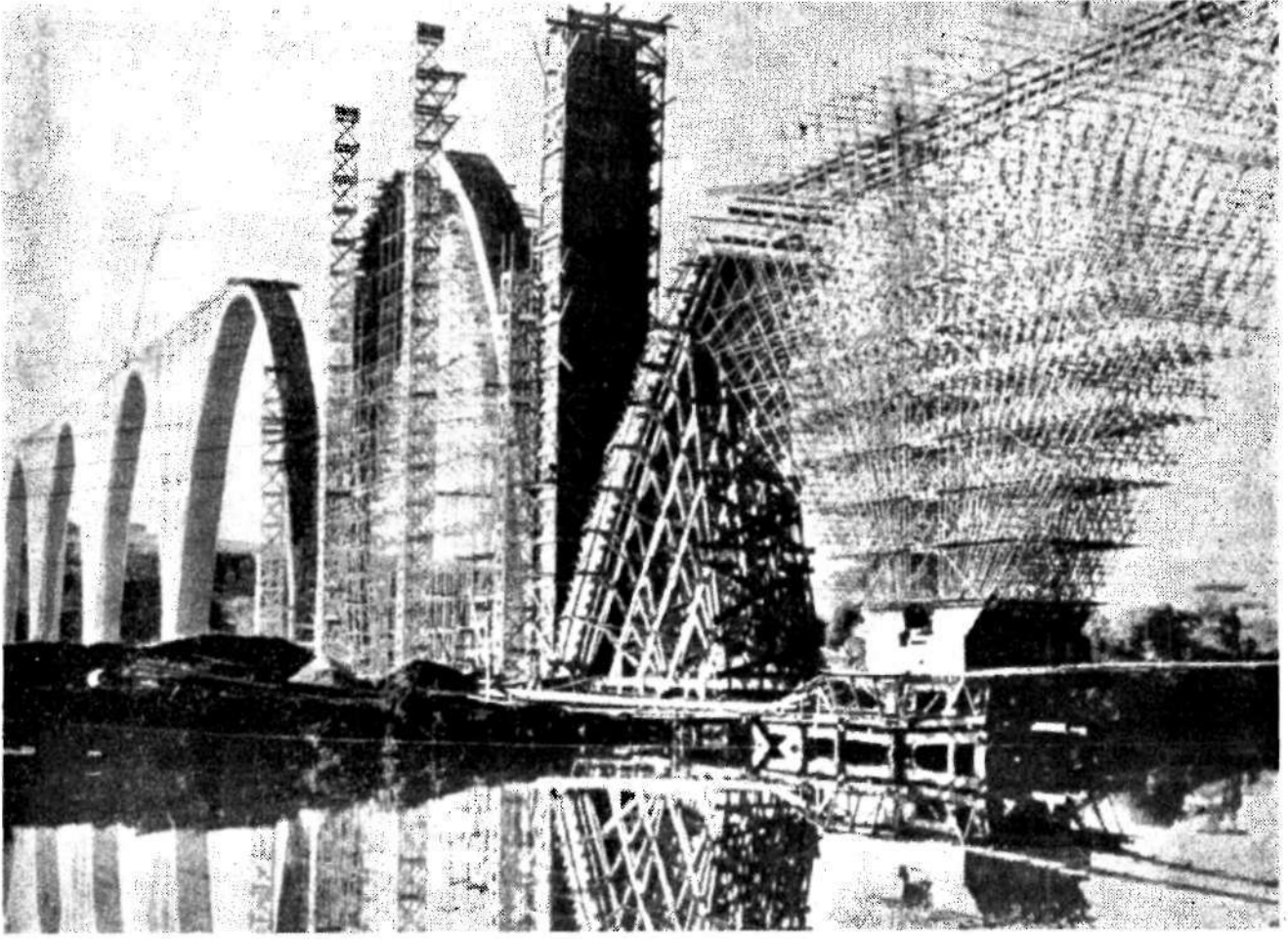
Brezilya'da «Papagaio» da yeni inşa olunan bir vladükün görünüşü.
