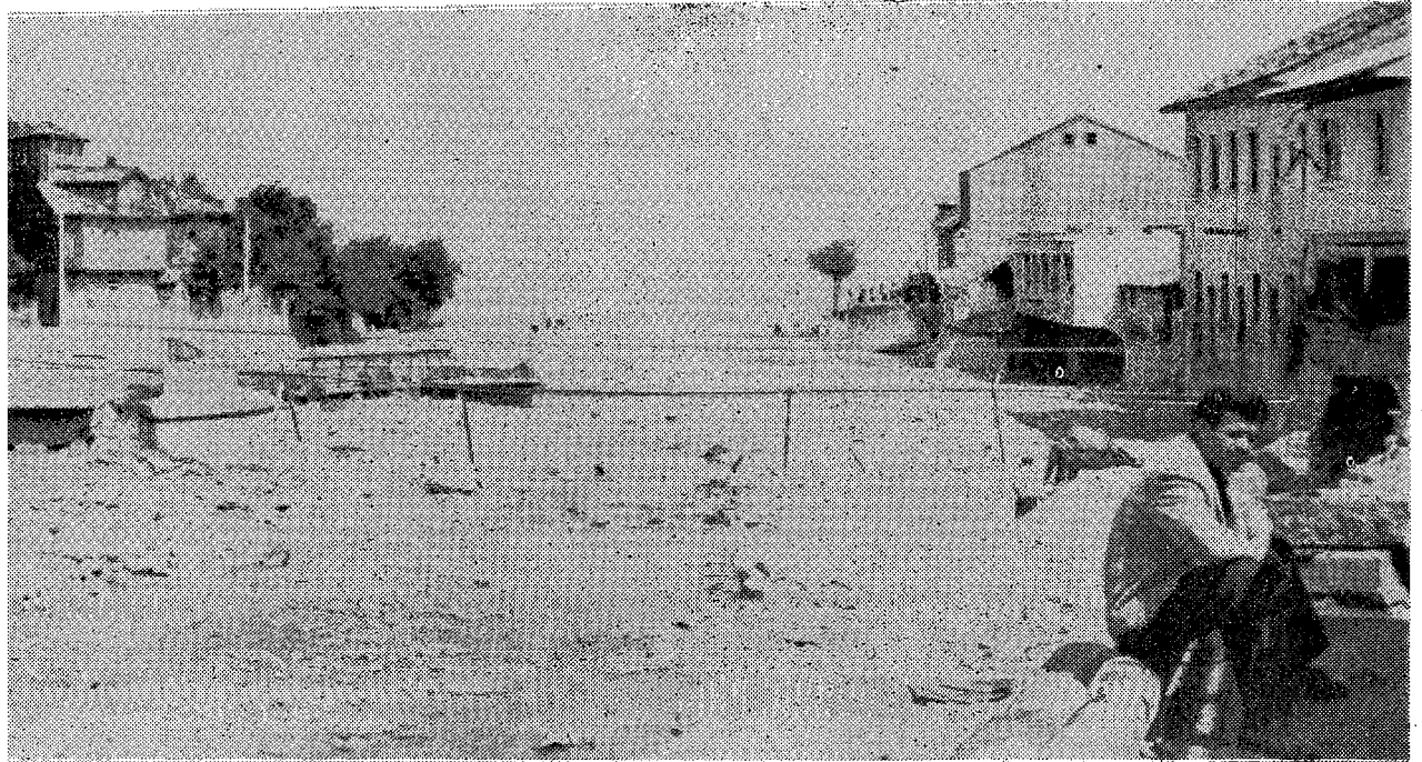
şolu Köprüsü — Akarsunun taşıdığı rusubat ve ağaçlar kesidi tıkayarak debuse yetersizliği köprünün yıkılmasına seep olmuştur. (Türkiye Mühendislik Haberleri)
