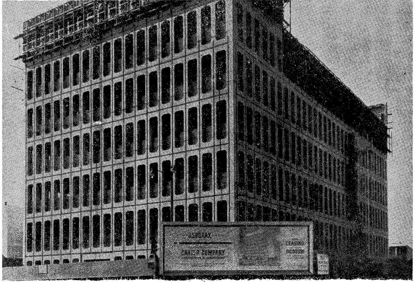
lik kalıplar üzerindeki konsollar bir üst katın kalıp iskelesi montajını kolaylaştırdığı için pahalı kalıp panoları aliyeti düşürüyor. (Engineering News - Record Nisan, 1963)
