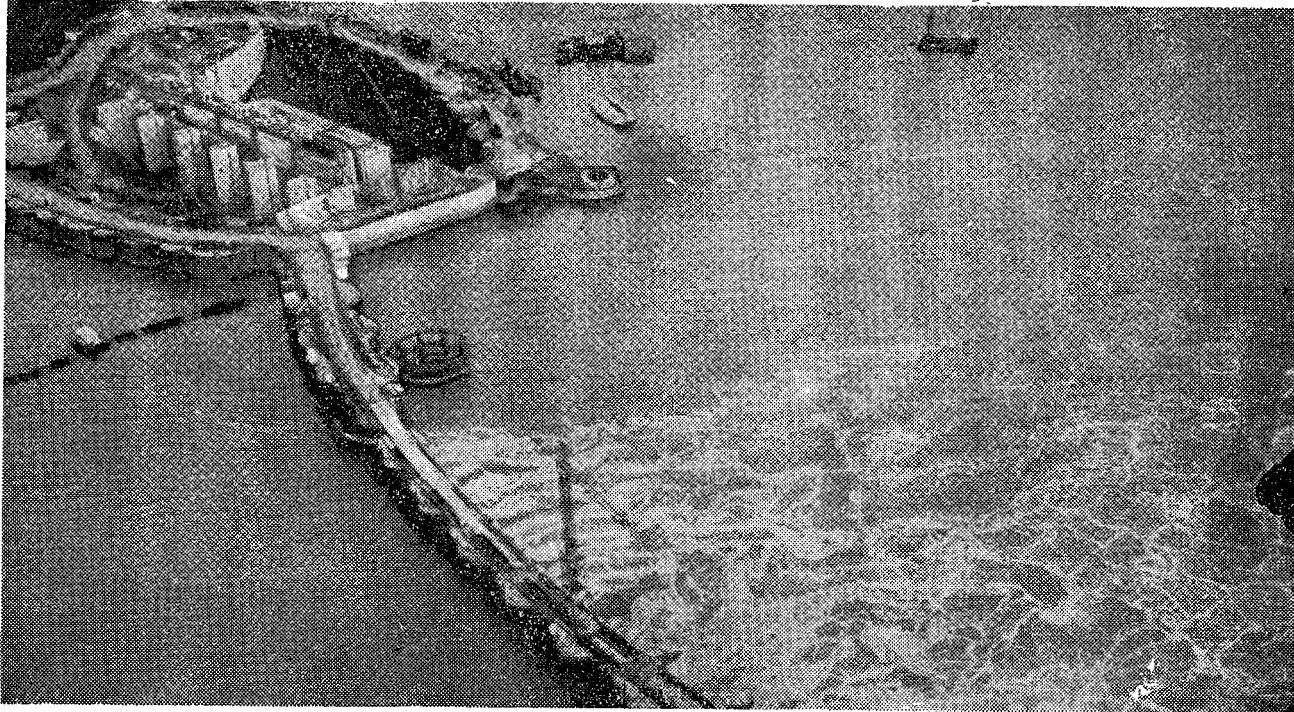
Met Suları Betonarme Kesonlar Arasından Akıyor. Kuleli Vinç ve Yolu Kesonlar Arasına Çelik Palplanş Çakma İşi İçin Hazırlanıyor. (Engineering News - Record. Nisan, 1963)
