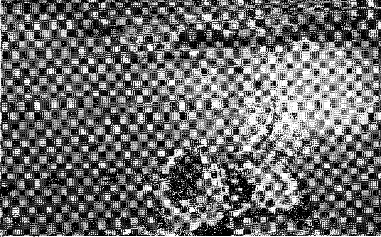
Rance Nehri Üzerinde Su Geçidini Kapatacak Olan Batordenun Mansap Duvarı İlerliyor. Nehrin Ortasında Sey. yar Basıncı Hava Kesonu Görülüyor. (Engineering News - Record. Nisan, 1963)
