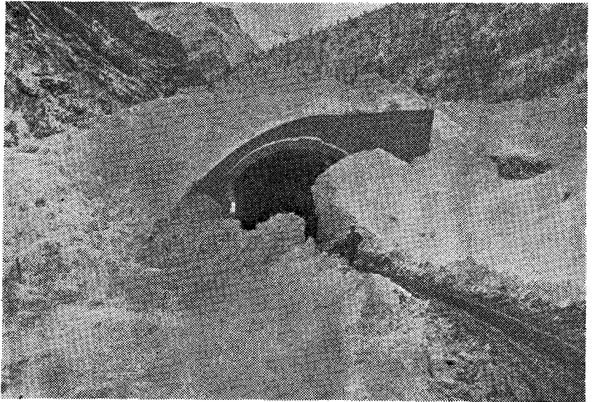
Resim 2 : km. 41+490—530 arasında inşa edilen çığ tünelinin, Pülümür ağzından görünüşü
