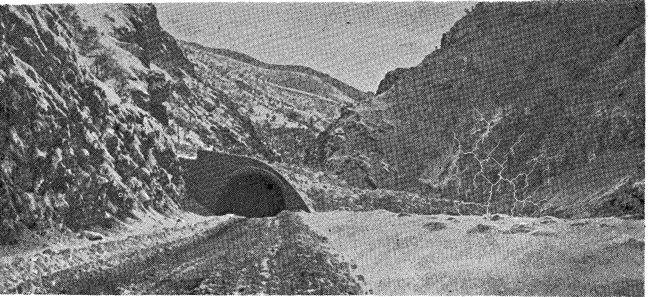
Resim 5 : km. 44+670—790 arasında inşa edilen çığ tünelinin (ki, bu tünel en uzun tölde olanıdır) Pülümür ağzından görünüşü.
