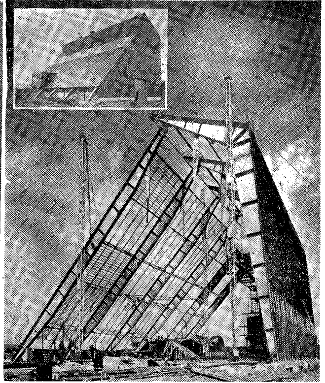
Fotoğrafi görülen tesis Fransa'da Paris banliyösünde MASSY - ANTONY termik santralının jeneratörlerini ihtiva etmektedir. Ultra modern olan bu bina, metalik şarpantın arduaz ile kaplanmasıyla inşa olunmuştur.
