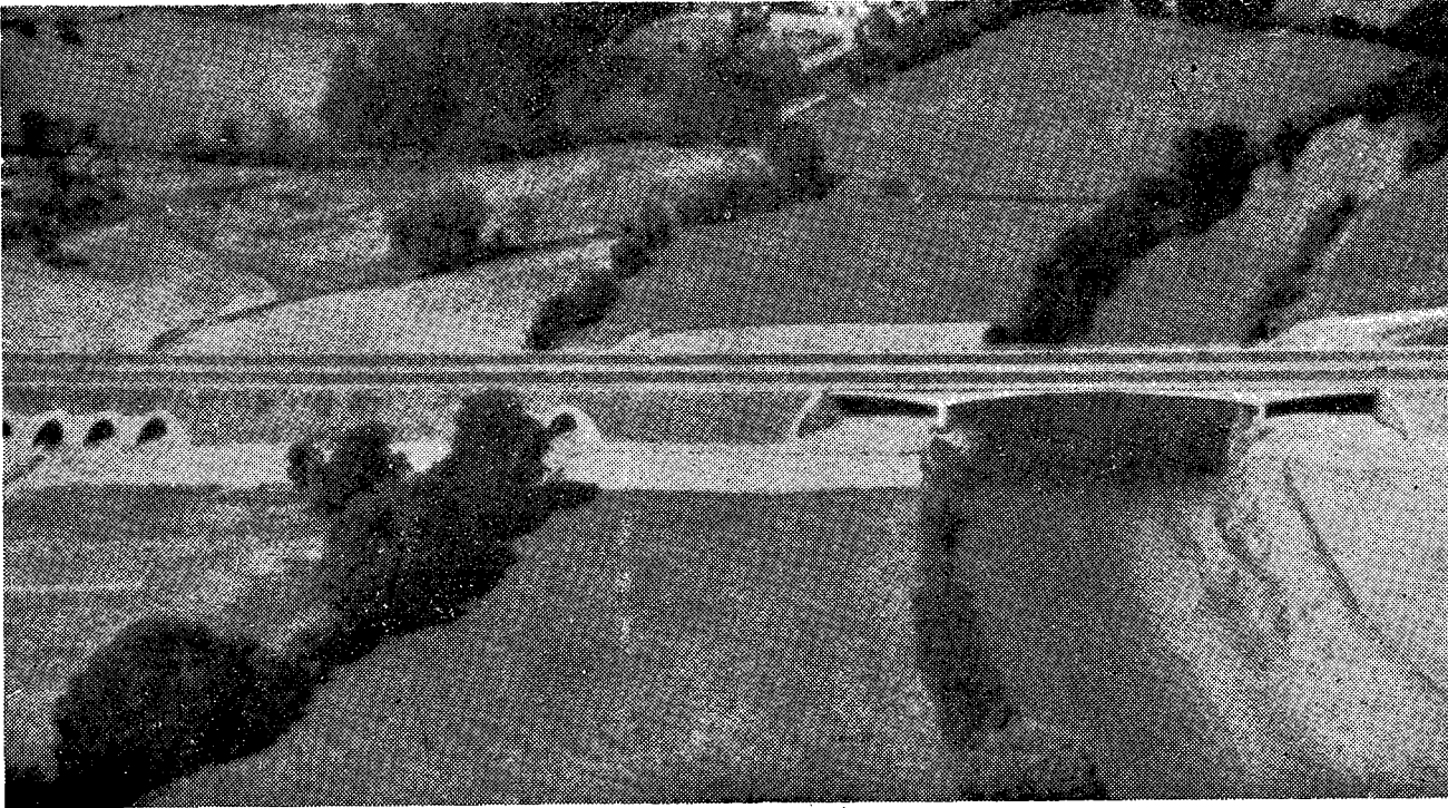
Bridstow kara yolu köprüsü (İngiltere) toplam uzunluk: 108 m. Orta açıklık: 62 m. Kenar açıklıklar: 23 m. Köprüyü betonarme diyaframlarla birbirine bağlı 9 ana giriş taşımaktadır
