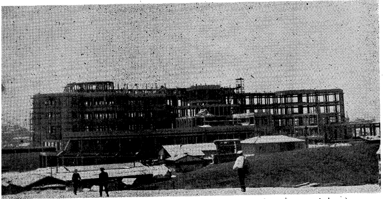
DİL-TARİH VE COĞRAFYA FAKÜLTESİ ARKASINDA (Hastahane İnşaatı - Ankara)
